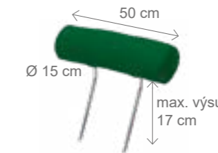
podhlavník ESTER
