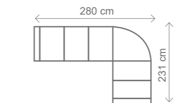
III. R (L) + R + II. ÚP (P) rozklad 205 x 123 cm
